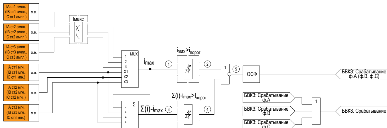
Рисунок 2.7 – Функциональная схема «БВКЗ»
